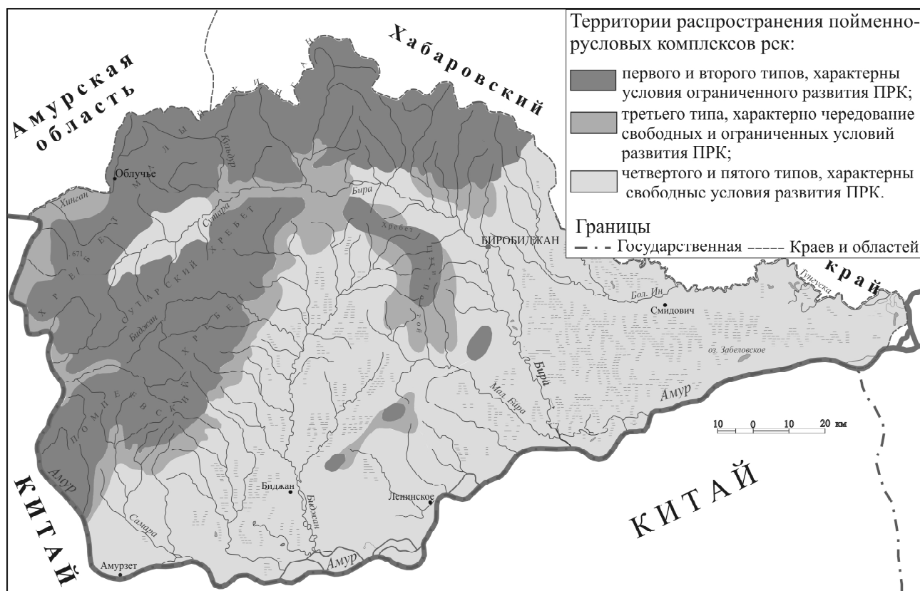
Рис. Зональность физико-географических условий развития пойменно-русловых комплексов рек Еврейской автономной области
